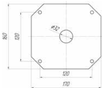
Рис.1. Геометрические размеры теплообменника
