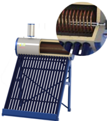
RPA-Теплообмен
